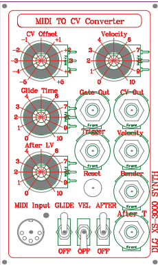
MIDI 2 CV
