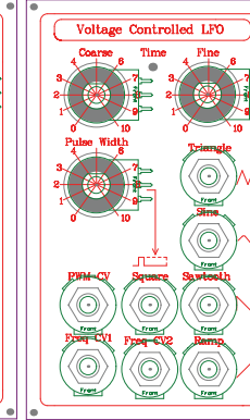
LFO
